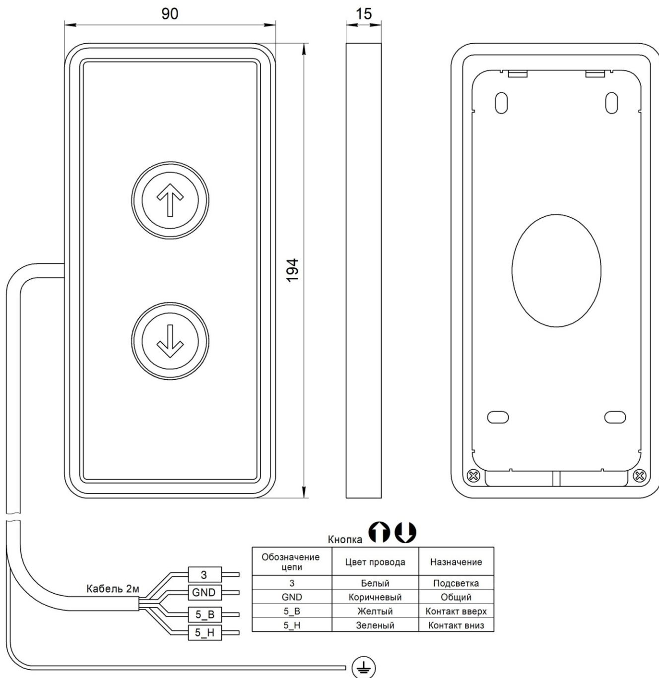
Рис.1 Внешний вид и габаритные размеры Вызывного поста ОБСИДИАН НШЕК.468381.225
